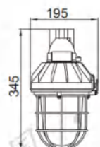
II 型 Type
