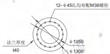
法兰平面示意图 Flange plane schemes
