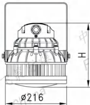
II型支架式
