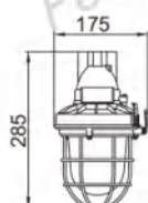
I 型 Type
