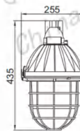
IV 型 Type
