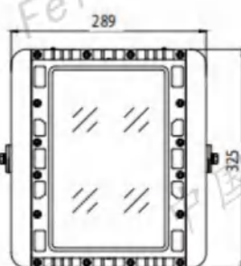
FCF(T)98-180W
