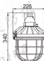
III 型 Type
