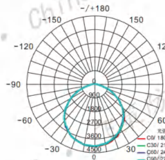
III型 Type
