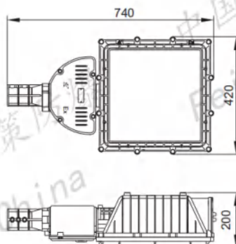
II 型/路灯一体式 II Type/Street lamp type/one-piece
