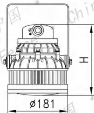
I型支架式
