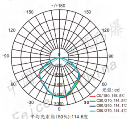
I 型 Type
