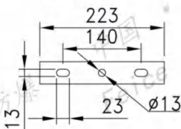
II型吸顶或壁式
