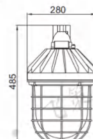
V 型 Type
