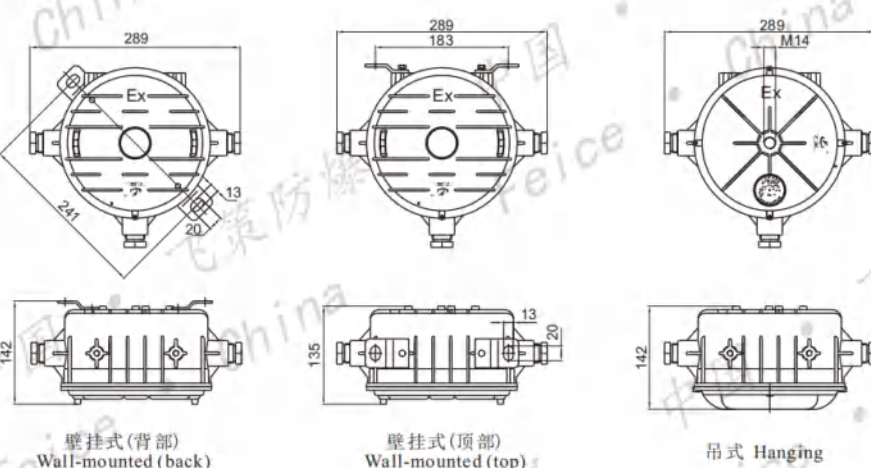
400W II 型
