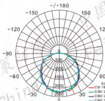
II型 Type
