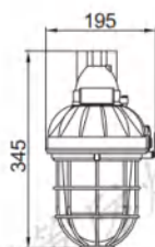
II 型 Type
