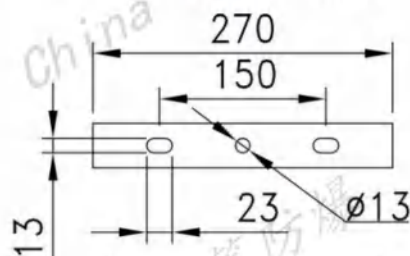
III型吸顶或壁式
