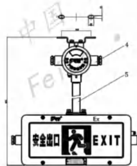
安装方式: 吊杆式 (G) Installation mode: boom type (G)
