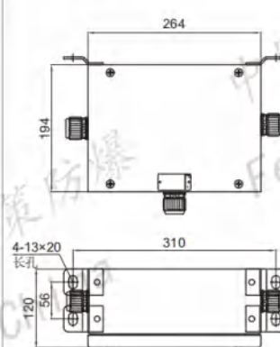
400W IV 型
