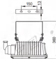
I 型 Type /分体式 red-tipped
