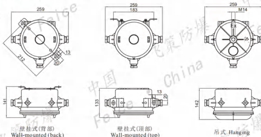
250W I 型
