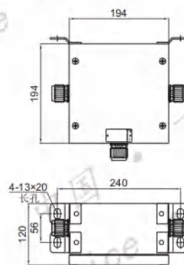
250W III 型
