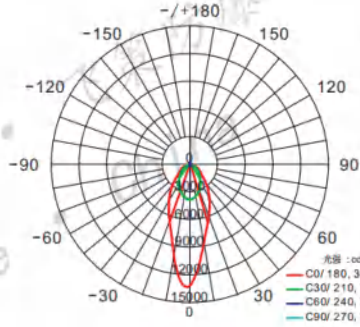
V型 Type
