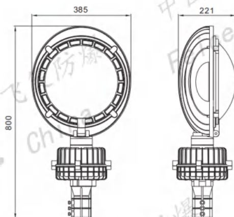
IV 型 Type
