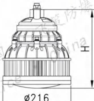
II型吸顶或壁式
