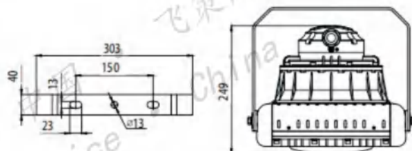
FCF98-120W
