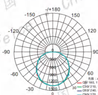
I 型 Type
