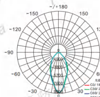
IV型 Type
