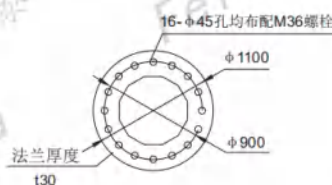
法兰平面示意图 Flange plane schemes
